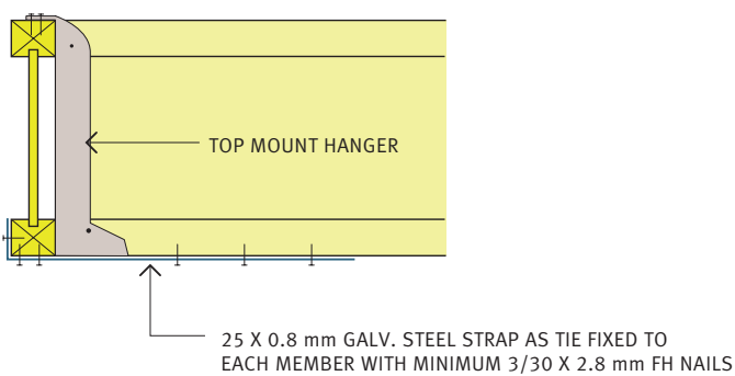
DETAIL F10
